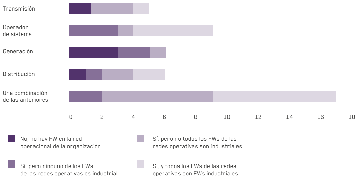
FIGURA 31. Uso de firewall en la red TO.
